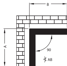
внутренний угол 90°
