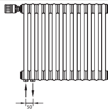
zehnder charleston completto Модель C 2050-12
