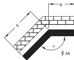
внутренний угол от 90° до 179°
