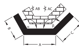
двойной внешний угол от 90° до 179°
